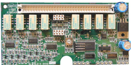
Kretskort, CT603
